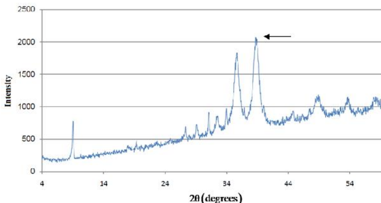
شکل ۳. نمونه الگوی پراش پرتوی ایکس (XRD) نانوذرات اکسید مس سنتزی
