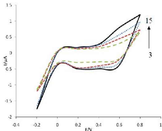
شکل ۵. منحنی‌های ولتاموگرام چرخه‌ای بدست آمده از الکتروود گلوکز اکسیداز اصلاح شده با نانوذره اکسید مس در محلول‌های گلوکز با غلظت‌های به ترتیب ۳، ۶، ۱۰، ۱۵ میلی مولار
