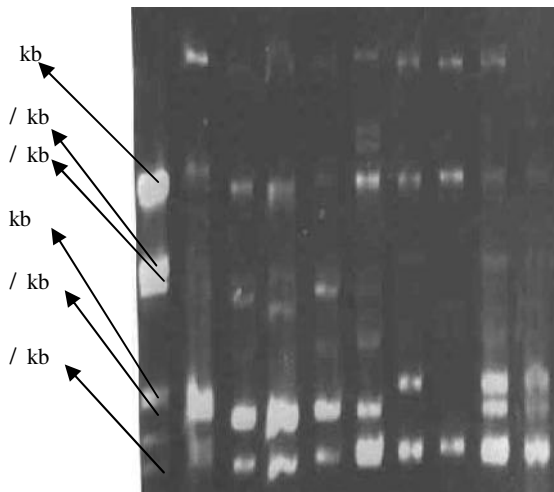
تصویر ۱. الکتروفورز DNA پلاسمیدی سویه های سودوموناس ترورینوزا ایزوله شده از بیماران مبتلا به عفونت زخم سوختگی در روی ژل آگارز ۰/۷٪. ستون های شماره (۳ و ۴) و (۹ و ۱۰) دارای الگوی پلاسمیدی مشابه و سایر ستون ها دارای الگوی پلاسمیدی متفاوت می باشند. خانه شماره ۱ مربوط به سایز مارکر DNA لامبدای هضم شده با آنزیم EcoRI و HindIII می باشد.
