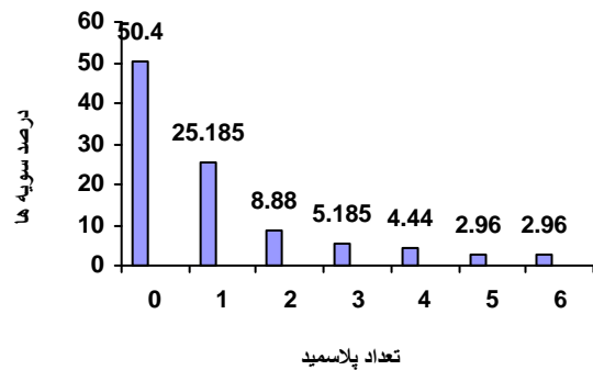
نمودار ۱. تعداد پلاسمیدهای ایزوله شده از سویه های سودوموناس آزمایشی
