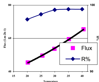
نمودار ۴. تغییرات راندمان حذف آرسنیک و فلاکس عبوری از غشاء RO با تغییر دمای محلول عبوری ( CAs = 0.2 mg/L، P = 225 psi، pH = 7 )
