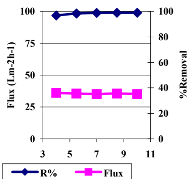
نمودار ۳. تغییرات راندمان حذف آرسنیک و فلاکس عبوری از غشاء اسمز معکوس TE ۲۵۲۱. با تغییر pH، CAs = 0.2 mg/L، P = 200 psi، (T = 20^\circ C)
