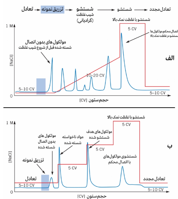
شکل ۹. کروماتوگرافی تعویض یونی [۱۶]
