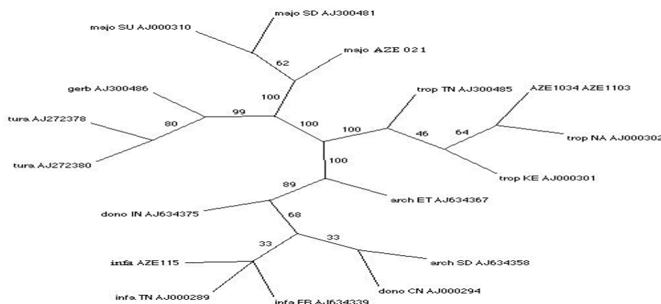
شکل ۲. درخت فیلوژنتیکی یک قطعه از ژن ITS1-5.8S- ITS2 شامل سه هاپلوتایپ از سه لیشمانیای جدا شده از پشه خاکیهای منطقه کلپیر به انضمام هاپلوتایپهای لیشمانیاهای بدست آمده از بانک جهانی ژن با استفاده از آنالیز parsimony analysis with branch-and bound Search و نرم افزار PAUP*
