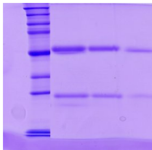
شکل ۳. ژل الکتروفورز برای بررسی صحت ساختار آواستین:
