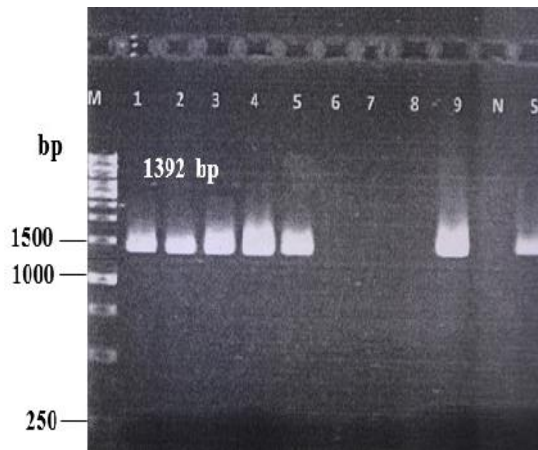
شکل ۶. شناسایی ژن phtE توسط PCR: M بیانگر مارکر وزن مولکولی، شماره ۱، ۲، ۳، ۴، ۵ بیانگر نمونه‌هایی از نتایج مثبت، N بیانگر کنترل منفی و S بیانگر نمونه کنترل مثبت (سویه استاندارد استرپتوکوکوس پنومونیه ATCC: 49619)
