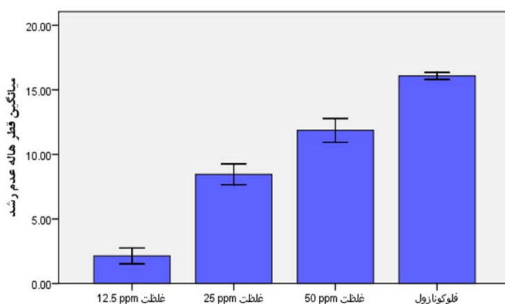
مودار ۲. میانگین قطر هاله عدم رشد در غلظت‌های ۵۰ ppm، ۲۵ و ۱۲/۵ از نانوذرات طلا و فلوکونازول (بر حسب میلی‌متر)
