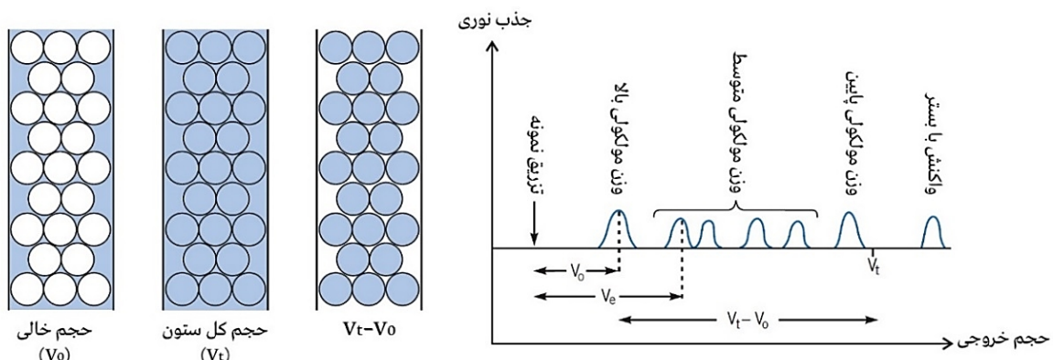
شکل ۴. نمودار هندسی V_0 و V_t عبارت V_t - V_0 شامل حجم مواد جامدی است که ماتریکس را تشکیل می‌دهد [۱۶]
