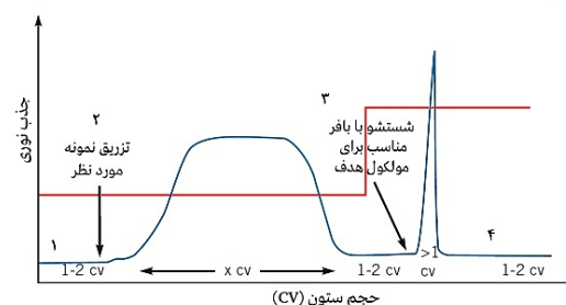
شکل ۱۱. تصویر شماتیک از کروماتوگرافی تمایلی و نمودار حاصل از آن
