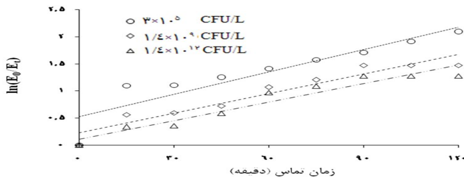
شکل ۴. سینتیک درجه یک بر روی کارایی حذف در سیستم فرابنفش (pH 7)
