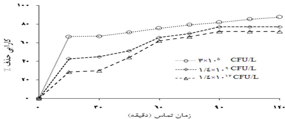
شکل ۳. تأثیر تعداد اولیه اشیریشیاکلی بر روی کارایی حذف در سیستم فرابنفش (pH 7)
