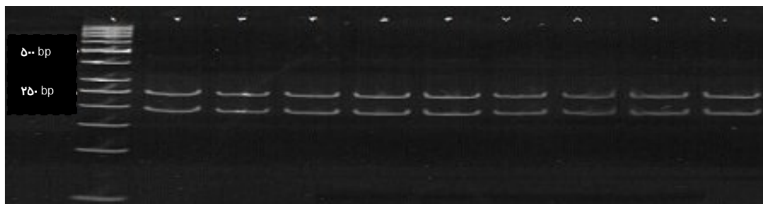
شکل ۲. محصولات برش با آنزیم Dde 1 بر روی ژل پلی آکریل آمید ۸٪. ستون ۱ مارکر مولکولی plus ۵۰ bp ، ستون ۹-۲ الگوی حساس دارای دو باند ۹۱، ۲۴۸ bp ، ستون ۱۰ سویه H37 RV است.
