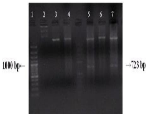
شکل ۲. هضم تک آنزیمی و دو آنزیمی با آنزیم های محدودالاندر پلاسمید (SacI, HindIII) بر روی ژل آگاروز (۱٪) چاهک ۱ و ۵: سایز مارکر (fermatas)، چاهک ۲: پلاسمید pET28a (+) نوترکیب بدون هضم آنزیمی، چاهک ۳ و ۴: پلاسمید pET28a (+) نوترکیب با هضم تک آنزیمی، چاهک ۵ و ۶: پلاسمید pET28a (+) نوترکیب با هضم دو آنزیمی
