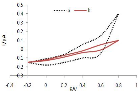
شکل ۴. ولتاموگرام چرخه ای الکتروکاتالیز گلوکوز اکسیداز اصلاح شده با نانوذره اکسید مس در حضور (a) و در غیاب (b) ۱ میلی مول گلوکوز در بافر فسفات
