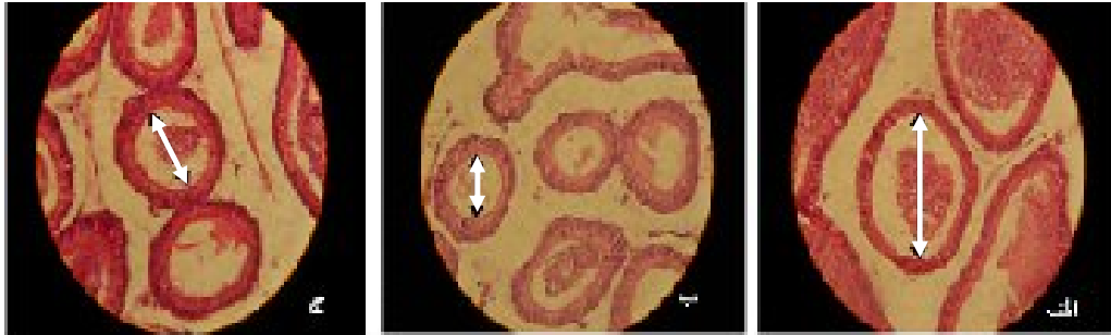
شکل ۱. تصاویر نشان دهنده مجاری اپیدیدیم با نمای میکروسکوپ نوری می باشند. الف: گروه کنترل که، مجرای اپیدیدیم با اپیتلیوم مطبق کاذب که دارای تعداد زیادی اسپرματοزئید در مرکز است، را نشان می دهد (پیکان). ب: گروه تحت استرس کم یک ماهه به کاهش قابل توجه قطر مجرای اپیدیدیم دقت کنید (پیکان). ج: گروه تحت استرس زیاد یک ماهه کاهش قطر مجرای اپیدیدیم مشاهده میشود (پیکان) (بزرگنمایی ۱۰).
